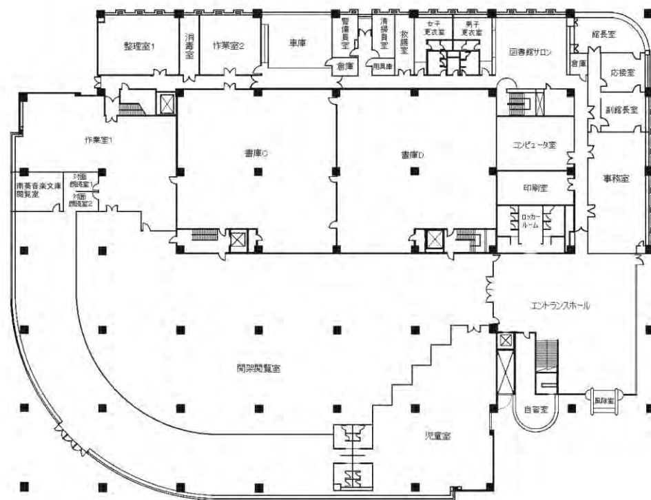
1F平面図
